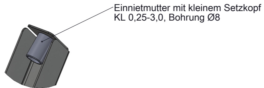
DETAIL F MAßSTAB 1 : 1
